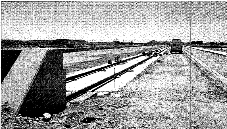
Estado que presenta el apartadero ferroviario que construye la sociedad TIM en el polígono "La Armentera". F.J.P.
